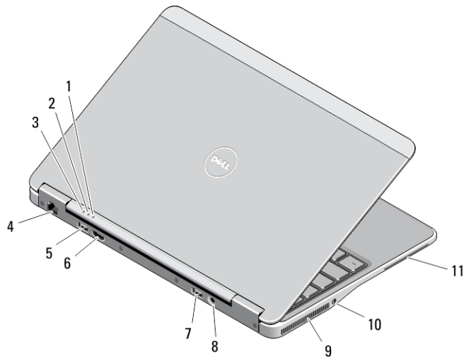
Abbildung 2. Rückansicht
